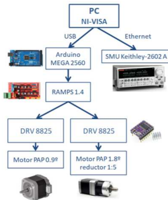
Figura 4: Esquema del hardware para controlar la base rotatoria y adquirir los datos.
