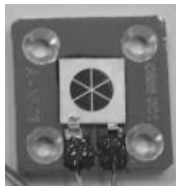
Figura 5: Sensor grueso de posición de ingeniería de la misión SAOCOM desarrollado en el DES.
